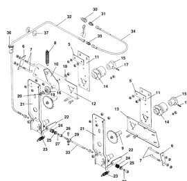
ETB-011715, Sprzęgło napędu
