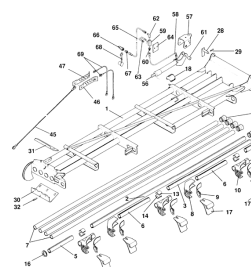
ETB-011705, Wysięgnik 16 m, lewy (1/2)
