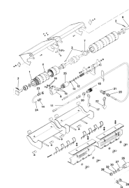
ETB-011762, Hydr. włączanie sekcji szerokości do mikrogranulatu, hydr. włączanie sekcji szerokości pr. (2/2)
