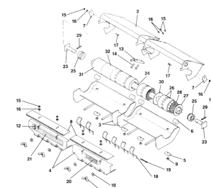
ETB-011741, Jednostka dozująca 9/7,5 do mikrogranulatu (jednostka dozująca lewa)
