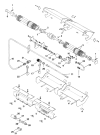
ETB-011756, Hydr. włączanie sekcji szerokości trzykrotne (2/2)
