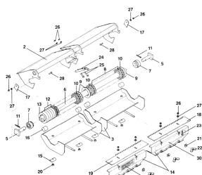
ETB-011735, Jednostka dozująca 10,5/8,75 do nawozu (jednostka dozująca prawa)
