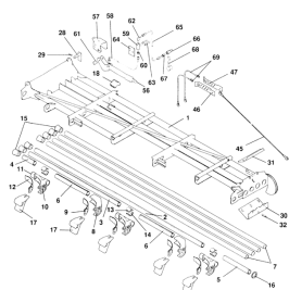
ETB-011703, Wysięgnik 15 m, prawy (1/2)
