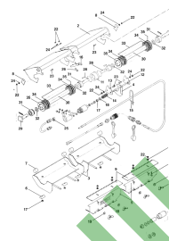
ETB-011757, Hydr. włączanie sekcji szerokości pięciokrotne (1/2)
