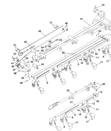
ETB-011702, Wysięgnik 15 m, lewy (2/2)
