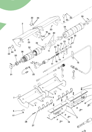
ETB-011761, Hydr. włączanie sekcji szerokości do mikrogranulatu, hydr. włączanie sekcji szerokości pr. (1/2)
