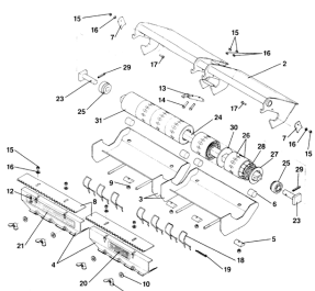
ETB-011739, Jednostka dozująca 10,5/8,75 do mikrogranulatu (jednostka dozująca lewa)
