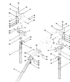
ETB-011730, Urządzenie do rozsiewu rzędowego - kolektor z tworzywa sztucznego
