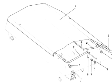
ETB-011761, Hydr. włączanie sekcji szerokości do mikrogranulatu, hydr. włączanie sekcji szerokości pr. (1/2)
