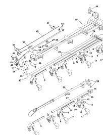
ETB-011706, Wysięgnik 16 m, lewy (2/2)
