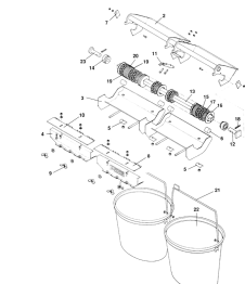
ETB-011718, Jednostka dozująca 15 m, lewa
