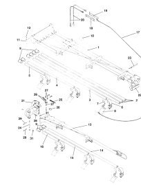
ETB-011698, Wysięgnik 10 m, prawy
