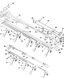
ETB-011712, Wysięgnik 18 m, prawy (2/2)
