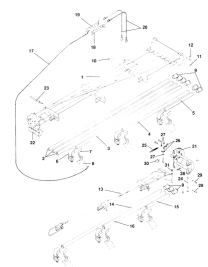
ETB-011699, Wysięgnik 12 m, lewy
