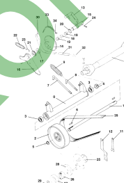
ETB-011713, Napęd, wersja F
