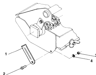
ETB-011744, Element dystansowy klap dennych
