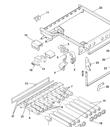
ETB-011726, Śluza iniektora 15 i 16 m, prawa
