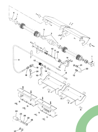
ETB-011760, Hydr. włączanie sekcji szerokości 5-krotne - nawóz - hydr. włączanie sekcji szerokości 5 le. (2/2)
