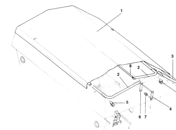
ETB-011762, Hydr. włączanie sekcji szerokości do mikrogranulatu, hydr. włączanie sekcji szerokości pr. (2/2)
