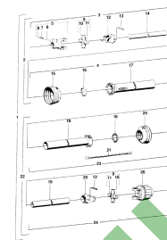
ETB-011745, Wałek przekąźnikowy 710 mm ze sprzęgłem jednokierunkowym
