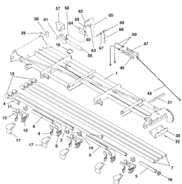
ETB-011707, Wysięgnik 16 m, prawy (1/2)
