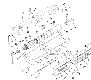
ETB-011742, Jednostka dozująca 9/7,5 do mikrogranulatu (jednostka dozująca prawa)
