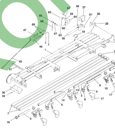
ETB-011701, Wysięgnik 15 m, lewy (1/2)
