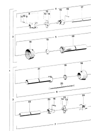
ETB-011729, Wałek przekątnikowy 710 mm
