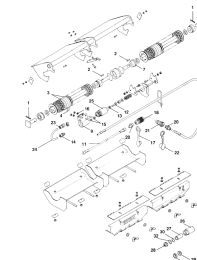
ETB-011754, Hydr. włączanie sekcji szerokości trzykrotne - nawóz - hydr. włączanie sekcji
