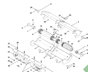
ETB-011736, Jednostka dozująca 9/7,5 do nawozu (jednostka dozująca lewa)
