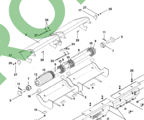
ETB-011737, Jednostka dozująca 9/7,5 do nawozu (jednostka dozująca prawa)
