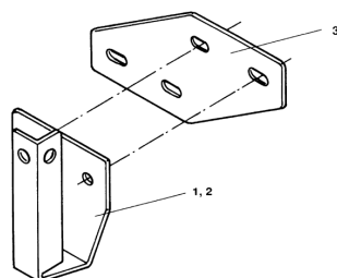
ETB-011747, Uchwyt tylnych świateł pozycyjnych kompl.
