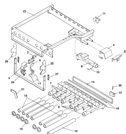
ETB-011724, Śluza iniektora 12 m, prawa
