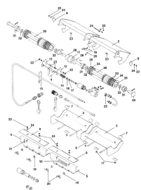
ETB-011755, Hydr. włączanie sekcji szerokości trzykrotne (1/2)
