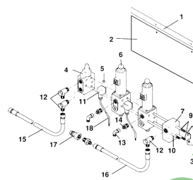
ETB-011748, Blok zaworowy dwukrotny
