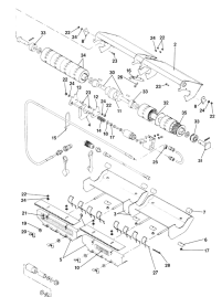
ETB-011759, Hydr. włączanie sekcji szerokości 5-krotne - nawóz - hydr. włączanie sekcji szerokości 5 le. (1/2)
