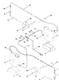
ETB-011733, Znacznik pianowy bez sprężarki
