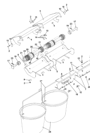
ETB-011717, Jednostka dozująca 10 i 12 m
