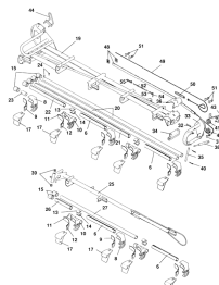
ETB-011708, Wysięgnik 16 m, prawy (2/2)
