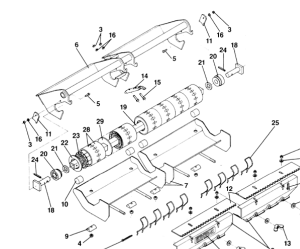
ETB-011734, Jednostka dozująca 10,5/8,75 do nawozu (jednostka dozująca lewa)
