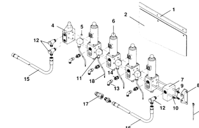
ETB-011750, Blok zaworowy czterokrotny
