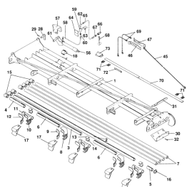
ETB-011711, Wysięgnik 18 m, prawy (1/2)
