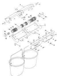
ETB-011719, Jednostka dozująca 15 m, prawa
