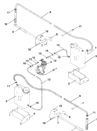
ETB-011732, Znacznik pianowy ze sprężarką
