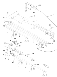
ETB-011700, Wysięgnik 12 m, prawy
