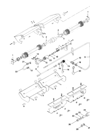
ETB-011758, Hydr. włączanie sekcji szerokości pięciokrotne (1/2)
