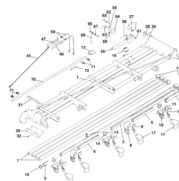
ETB-011709, Wysięgnik 18 m, lewy (1/2)
