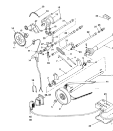
ETB-011714, Napęd, wersja H (zestaw doposażeniowy)
