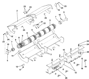
ETB-011743, Jednostka dozująca do nasion traw
