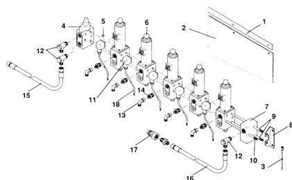
ETB-011751, Blok zaworowy pięciokrotny
