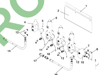
ETB-011749, Blok zaworowy trzykrotny
