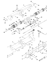
ETB-011753, Hydr. włączanie sekcji szerokości trzykrotne
